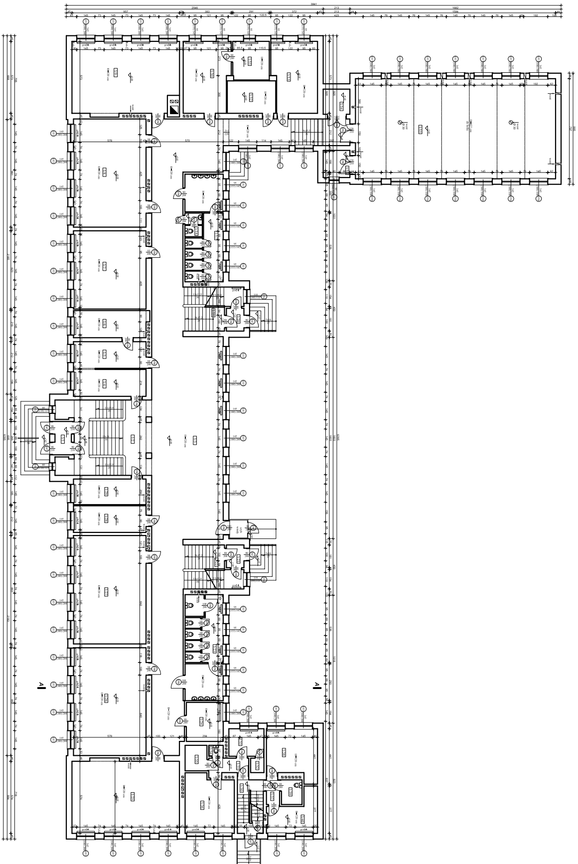
RZUT PARTERU 1:100
